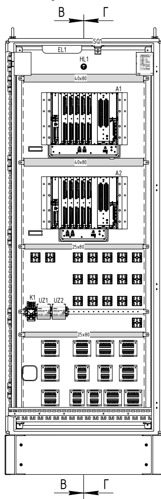
Рисунок В.2 – Чертеж общего вида (часть 2)
