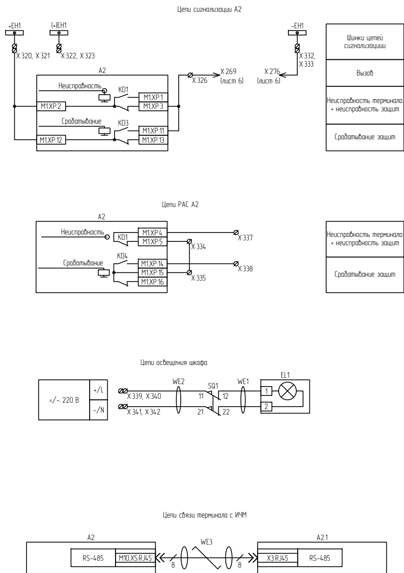
Рисунок Г.9 – Схема электрическая принципиальная (часть 9)
