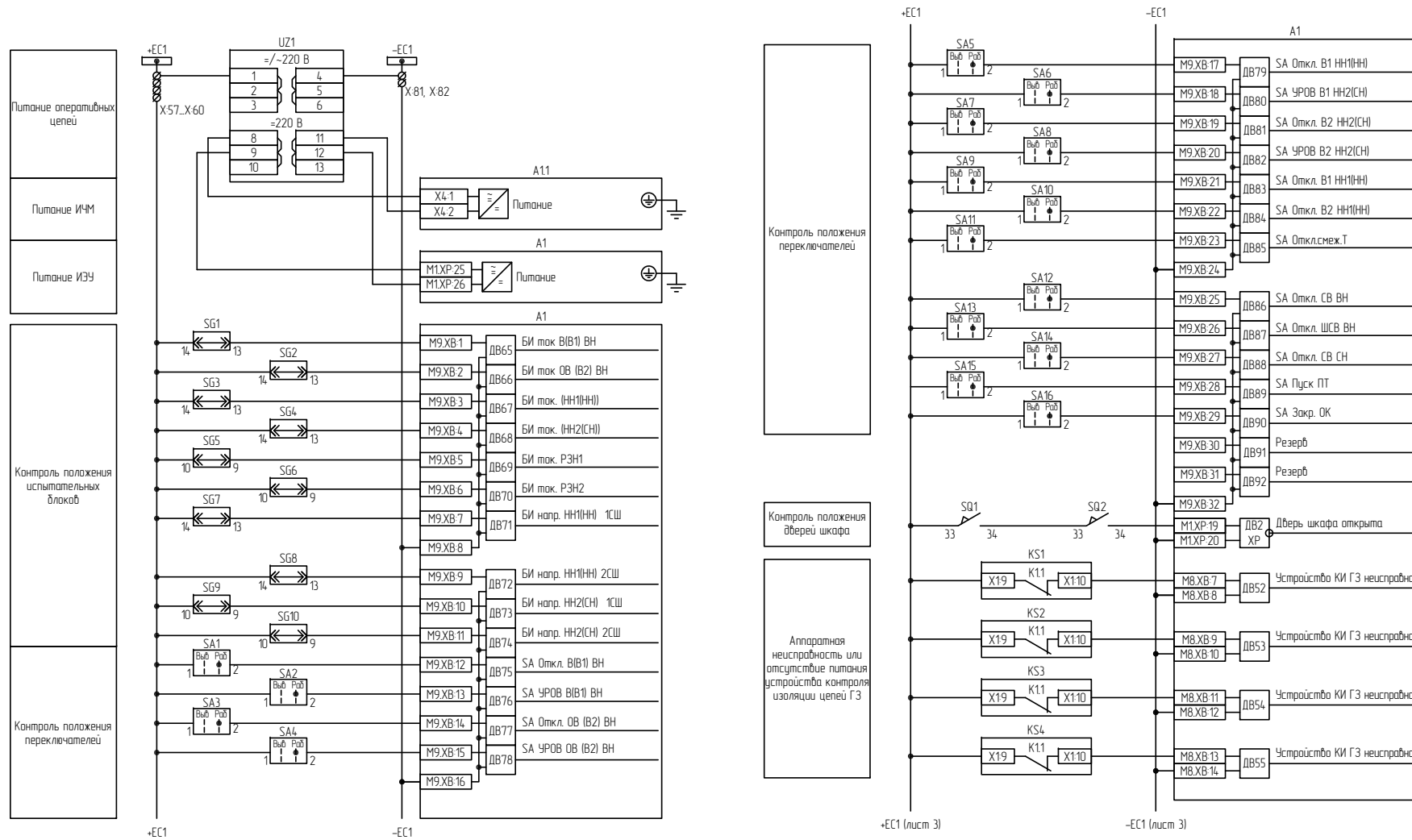
Цепи оперативного тока А1
